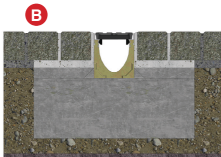
Pose en chaussée pavée
