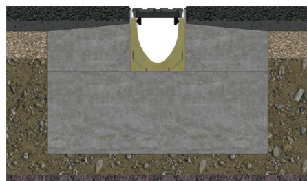
Pose en chaussée asphaltée ou enrobée
