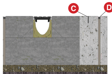
Pose en chaussée béton
